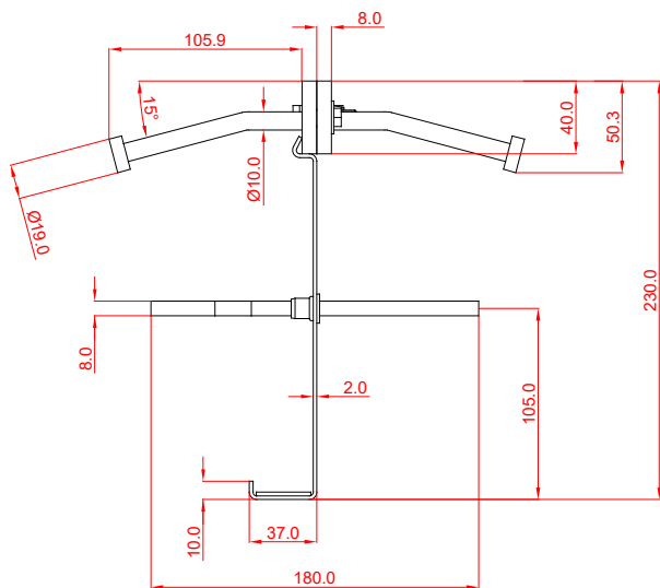
SEZIONE SCALA 3:1
