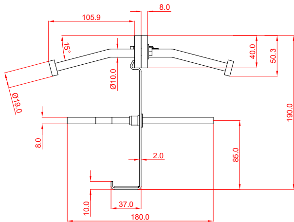
SEZIONE SCALA 3:1
