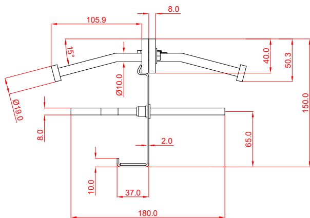
SEZIONE SCALA 3:1
